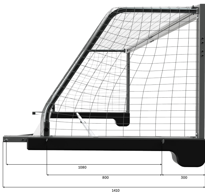
Målets mått med förlängare-kit Art. nr. 1514037
